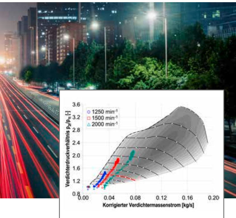
Bewertung von Lastsprüngen im Verdichterkennfeld
